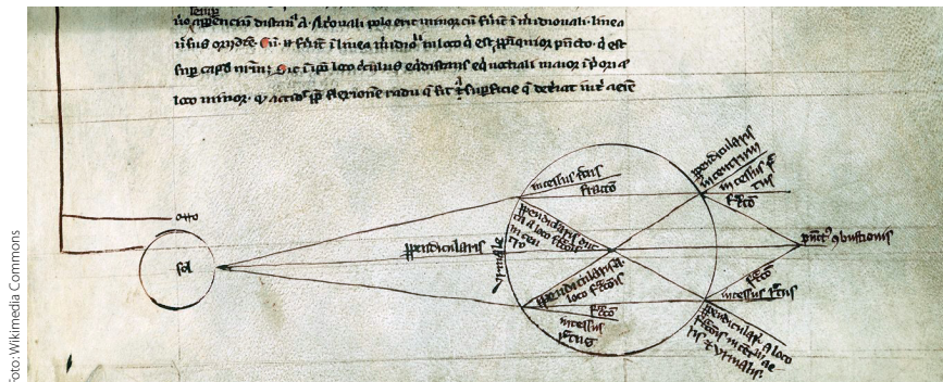
Digram z Baconova spisu „Opus maius“ ukazuje, jak se lámou sluneční paprsky
